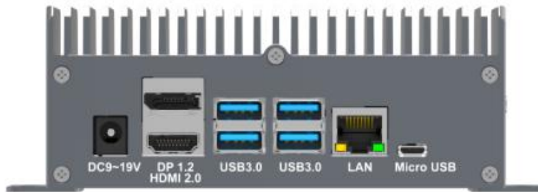
正面接口示意图
