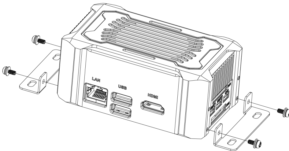
安装盒子支架
